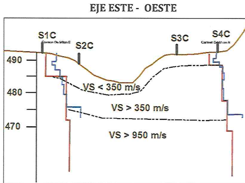
Perfil geofísico ortogonal a la líneas entrada 1 y salida 1. En azul V_s de MASW, en rojo V_s de REMI.
